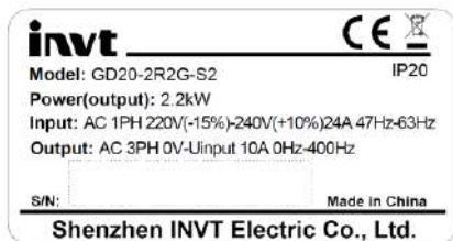
Рис. 2-1 Шильдик ПЧ
